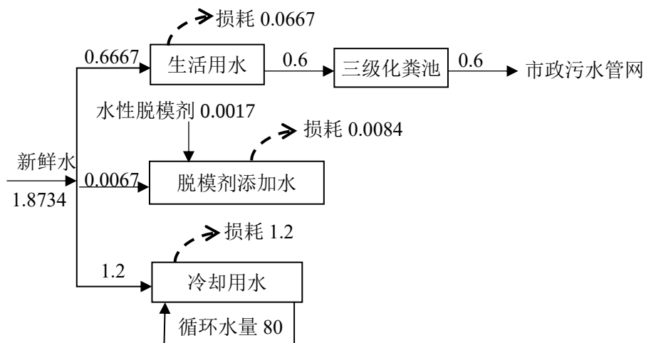
图2-1 项目水平衡图（单位：t/d）
