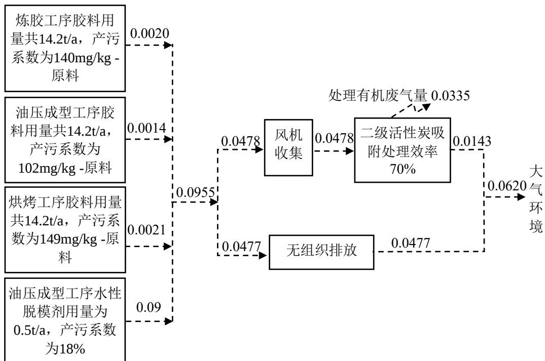
图 2-2 项目挥发性有机物平衡图 (单位: t/a)
