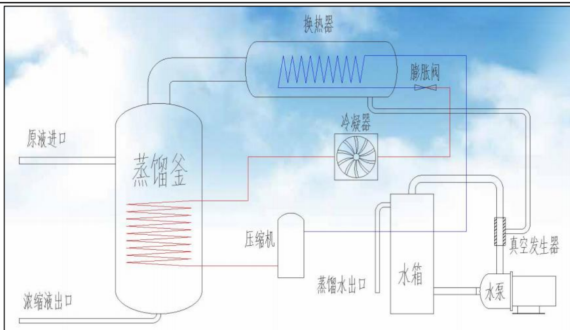
图4-2 低温蒸发器设备原理图
