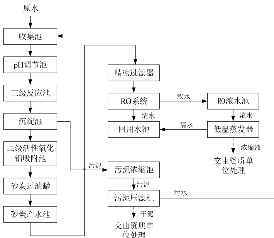
图4-1 项目生产废水处理工艺流程图
