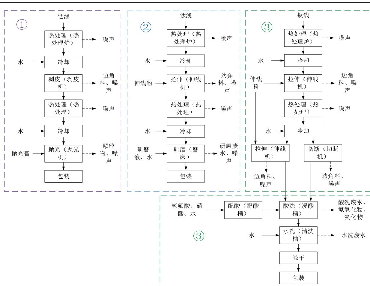
图2-2 钛线加工生产工艺流程图
