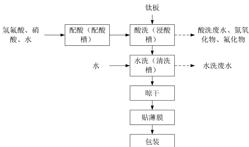
图2-3 钛板加工生产工艺流程图
