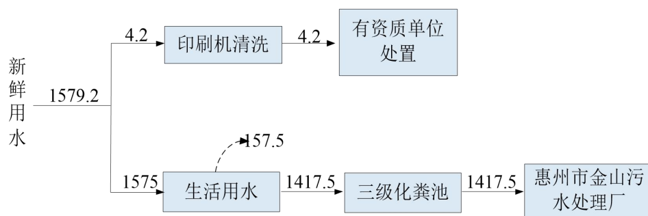
图 2 项目水平衡示意图 单位：m³/a
