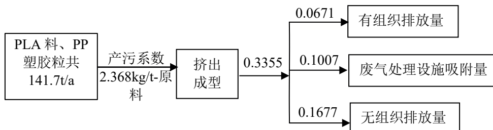
图 2-2 项目 VOCs 平衡图 (单位: t/a)
