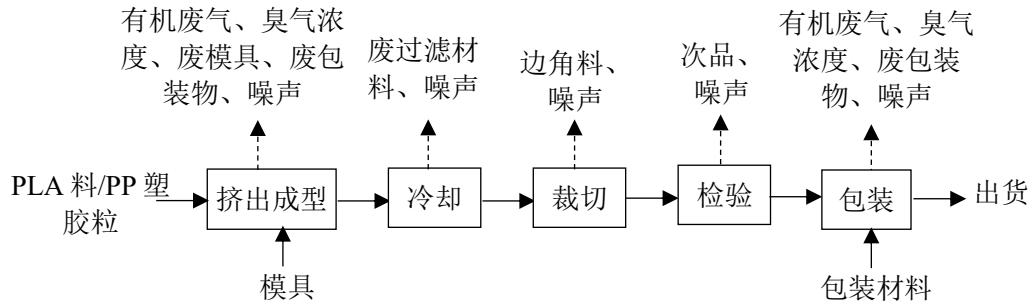
图 2-3 项目吸管生产工艺流程图及产污环节示意图
