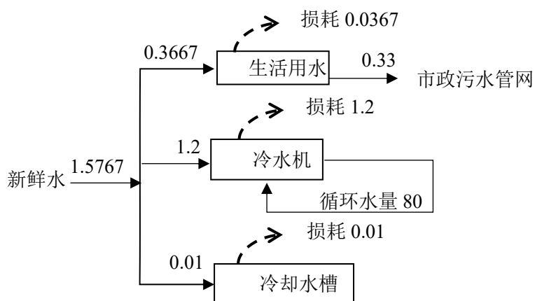
图2-1 项目水平衡图 (单位: t/d)
