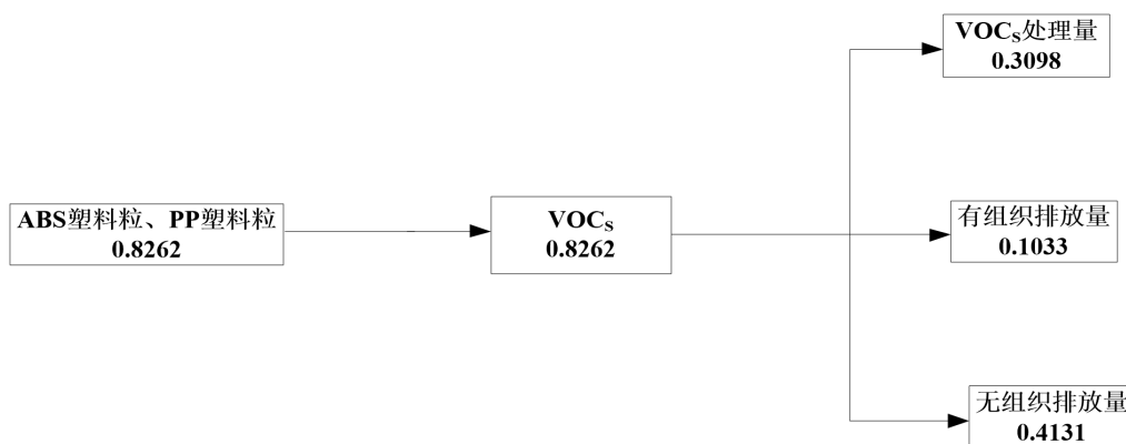
图2-1 项目VOCs平衡图t/a
