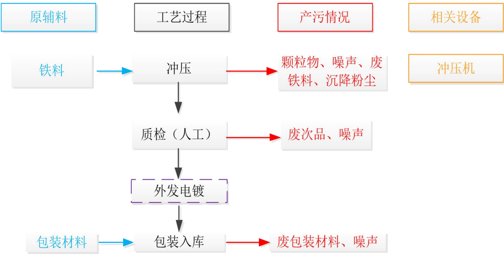
图 2-4 本项目五金零件生产工艺流程图
