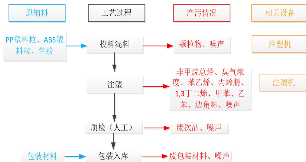
图 2-3 本项目塑料零件生产工艺流程图
