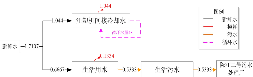
图2-2 本项目水平衡图（吨/日）
