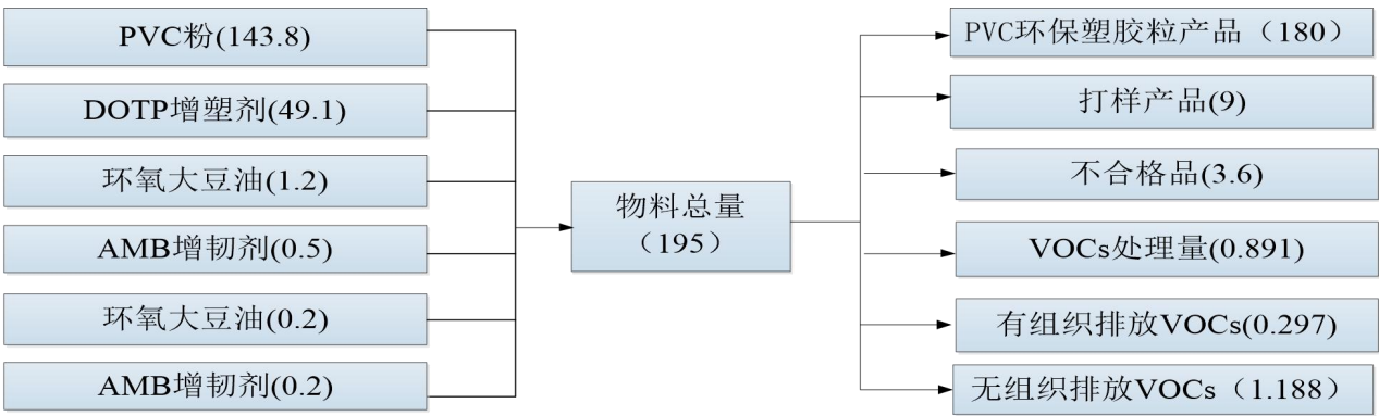
图 2-1 项目 VOCs 平衡图 单位：t/a
