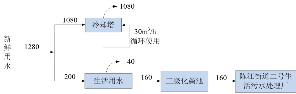
图 2-1 迁扩建项目水平衡图 (t/a)
