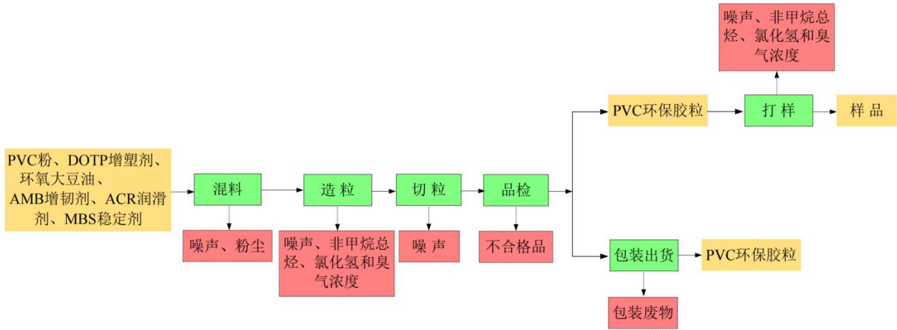
图 2-2 迁扩建项目 PVC 环保塑胶粒产品工艺流程及产污环节分析图
