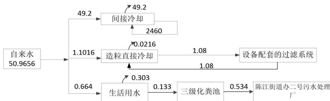
图 1 本项目水平衡图 单位：t/d
