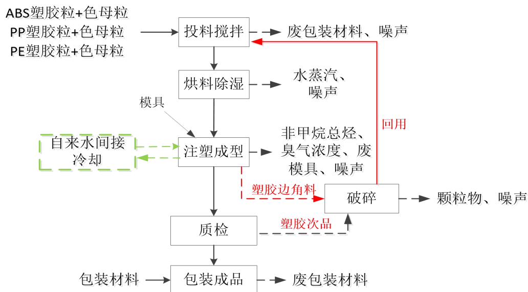
图 4 喇叭壳生产工艺流程图
