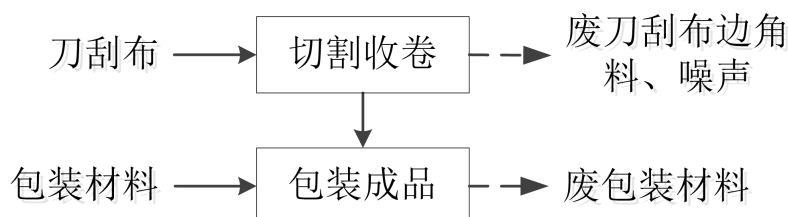
图 3 刀刮布生产工艺流程图
