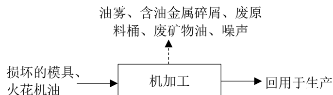
图 2-6 模具维修工艺流程图
