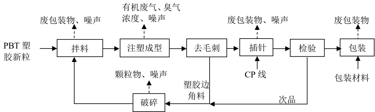
图 2-4 变压器骨架 1#生产工艺流程及产污环节示意图
