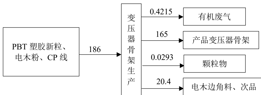
图2-2项目物料平衡图 (单位: t/a)
