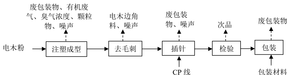
图 2-5 变压器骨架 2#生产工艺流程及产污环节示意图
